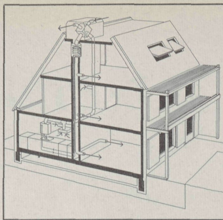
■ Een opengewerkte tekening van de huizen met ventilatiesysteem, luiken, passieve zonne-energie etc.
