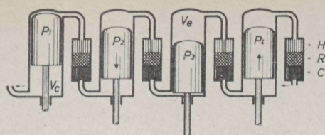
■ Schematische voorstelling van een dubbelwerkende viercilinder-Stirlingmotor. De symbolen hebben dezelfde betekenis als in fig. 13. Het open uiteinde rechts onder C, moet aangesloten gedacht worden op de opening links van de linkercilinder. Er zijn hier geen aparte zuigers en verdringers; de expansieruimte van de ene cilinder staat via H, R en C in verbinding met de compressieruimte van de volgende.
