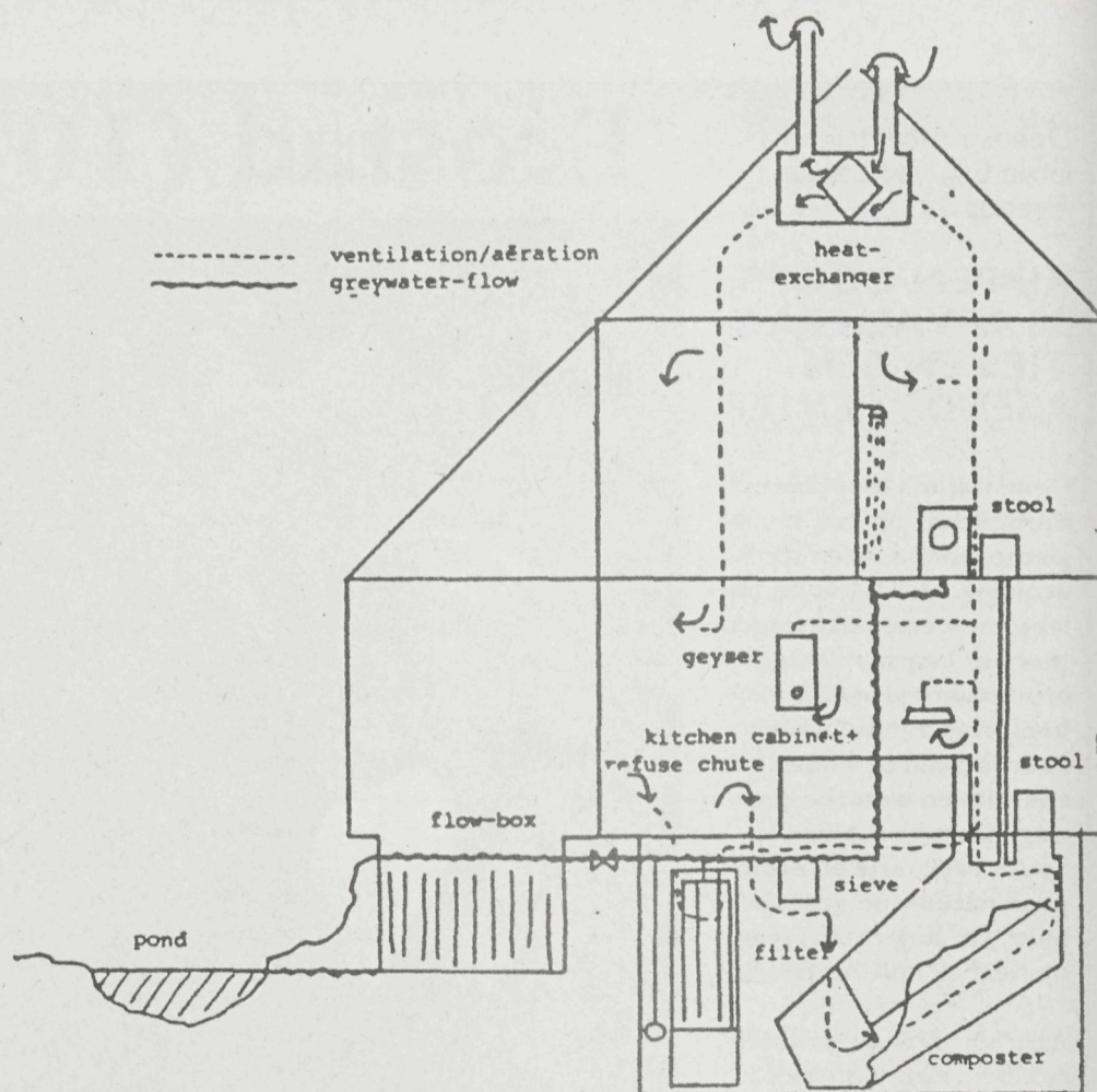
Het huis van De Man in doorsnee
