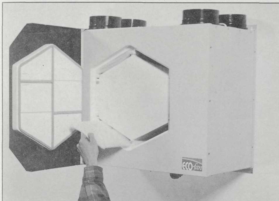
Warmteterugwin-unit (Itho)
